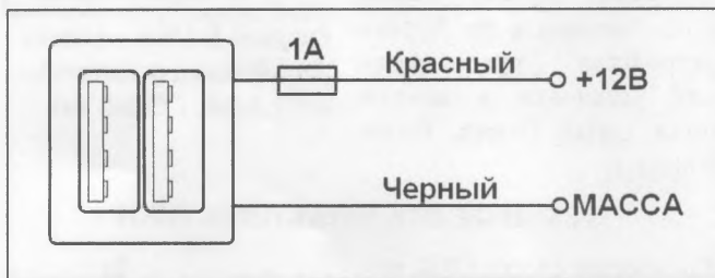
Рисунок 2. USB зарядное устройство для автомобилей LADA. Схема подключения
